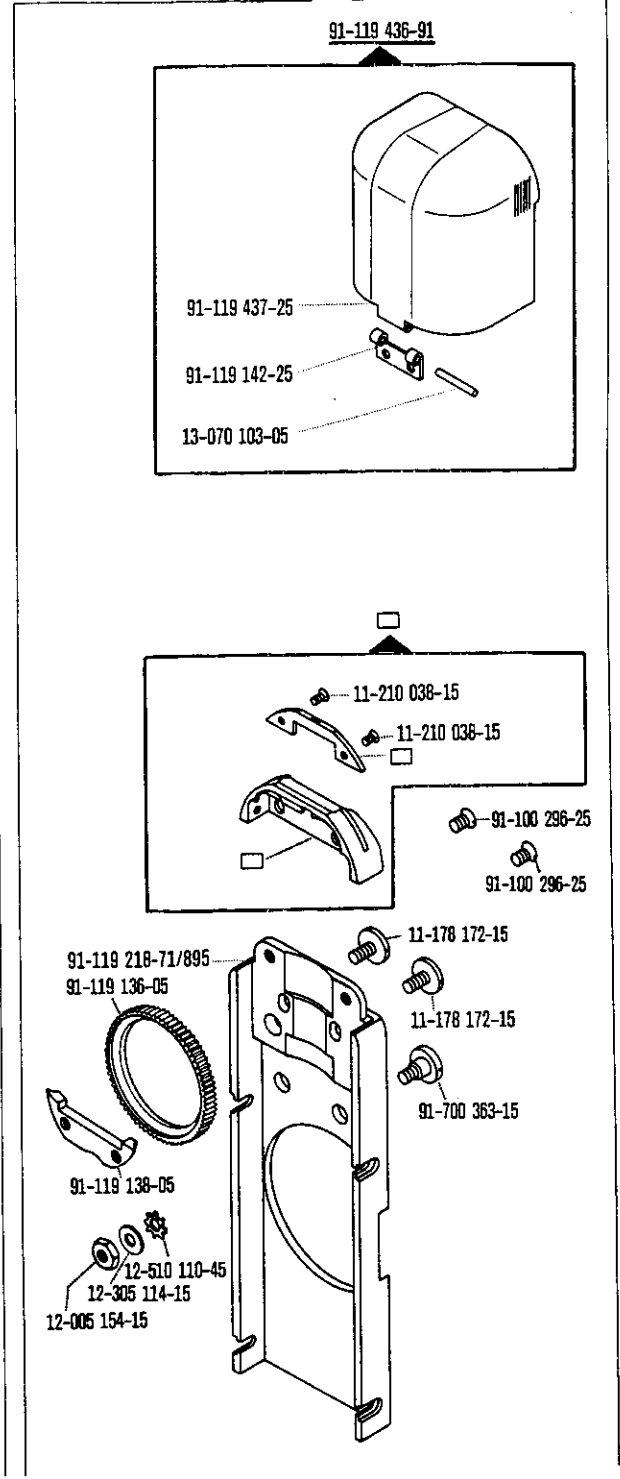
Pfaff 471-755/11-940/02
