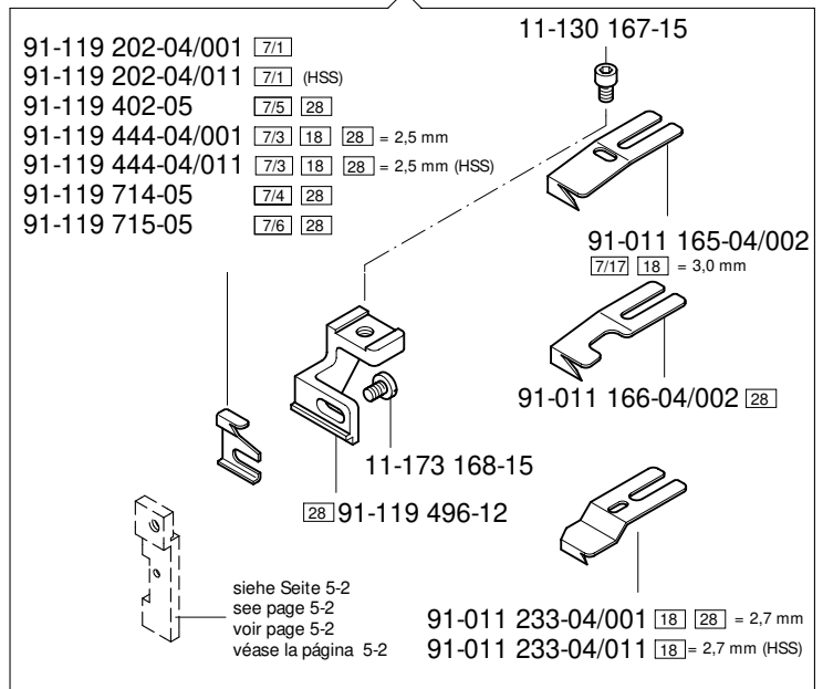
(PFAFF 471)
