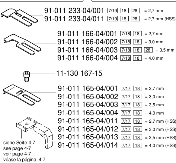
(PFAFF 471)
